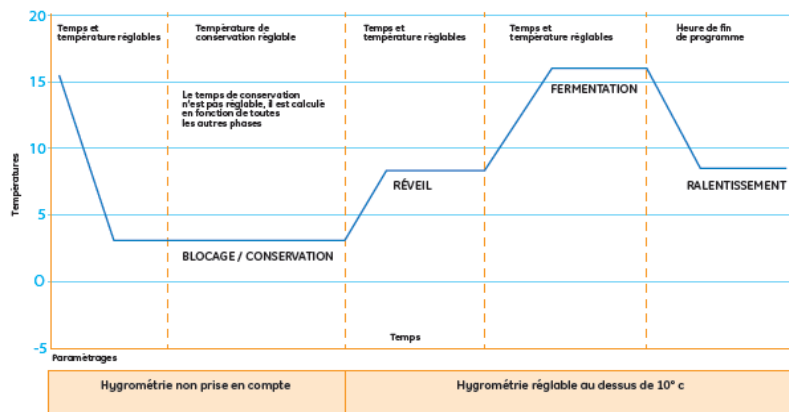
SYNOPTIQUE D'UN CYCLE AUTOMATIQUE
